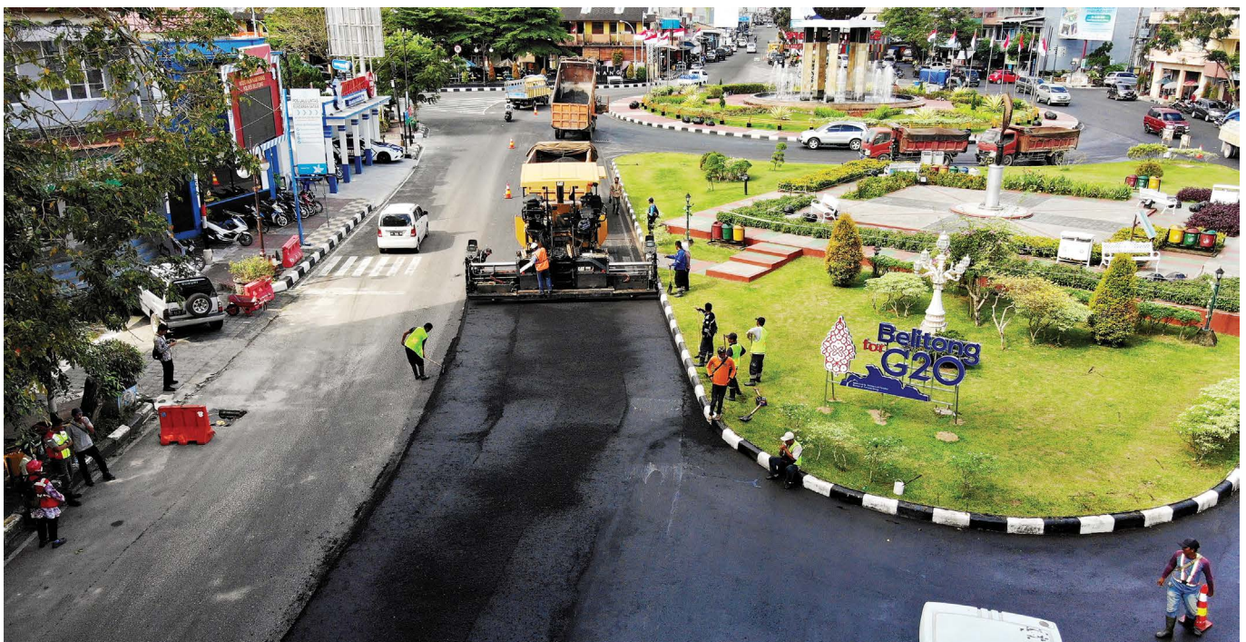
Pelaksanaan overlay HRS-WC di Bundaran Tugu Satam, salah satu ikon Kota Tanjungpandan.
